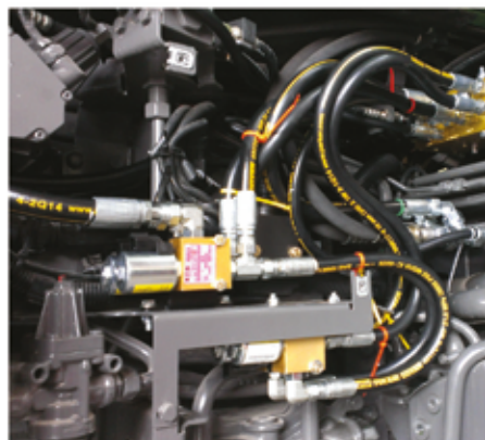
Direkter Eingriff in die Lenkhydraulik
