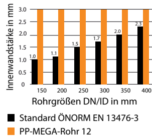
Innenwandstärkenvergleich
