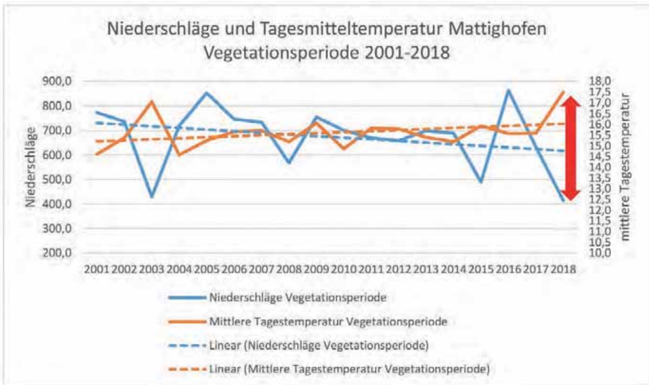
Diagramm 2: Niederschläge und Tagesmitteltemperaturen Mattighofen, Vegetationsperiode 2001-2018; Peter Frühwirth, nach Daten des Hydrografischen Dienstes OÖ.
