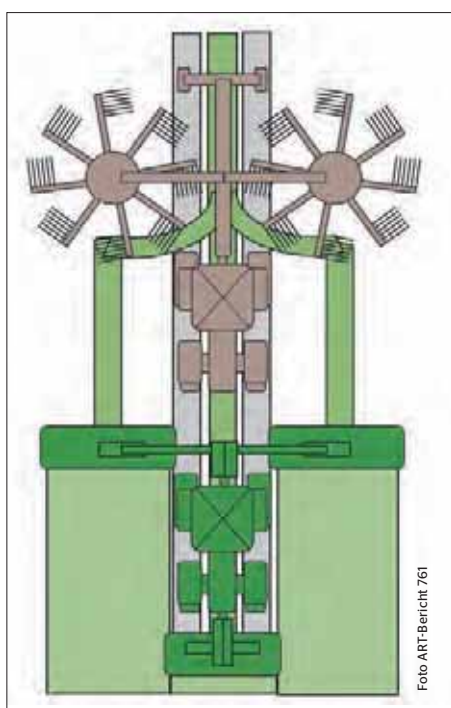
Traktorbasierte Grünlandkette mit 9 m Arbeitsbreite. Der Spurflächenanteil sinkt auf 13%.
