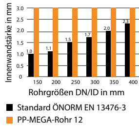
Innenwandstärkenvergleich
